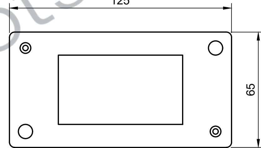
BOTTOM (OD)
