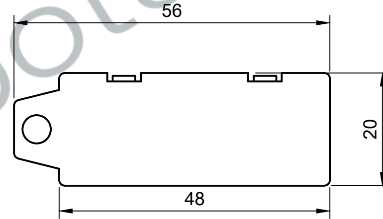
BOTTOM(OD)
