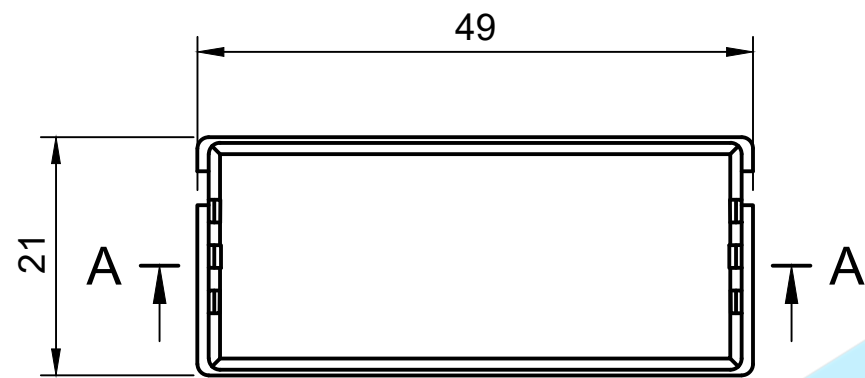
TOP(OD)
